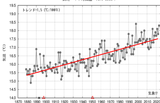
長崎 年平均気温 1879-2023年
