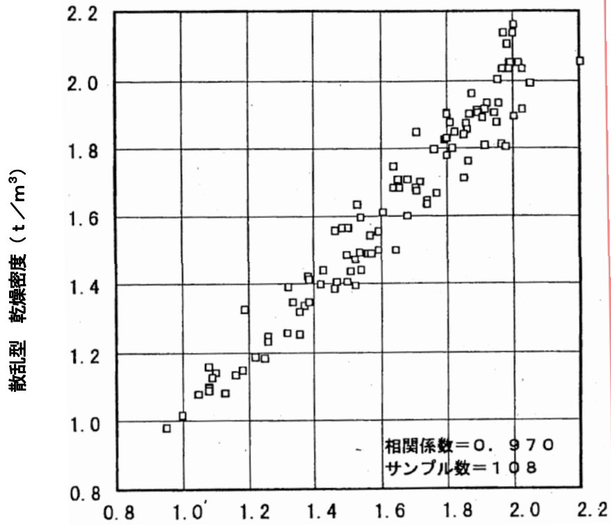
砂置換 乾燥密度 ( t/m^3 ) 図一 砂置換と散乱型の相関 (乾燥密度・全データ)
