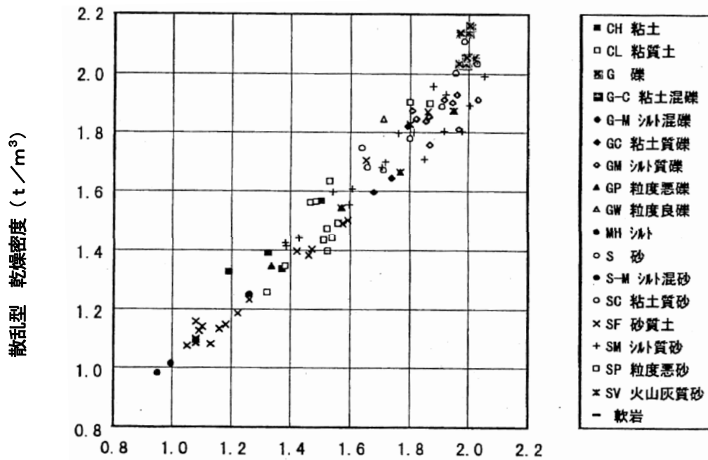
砂置換 乾燥密度 ( t/m^3 ) 図二 砂置換と散乱型の相関 (乾燥密度・土質別データ)
