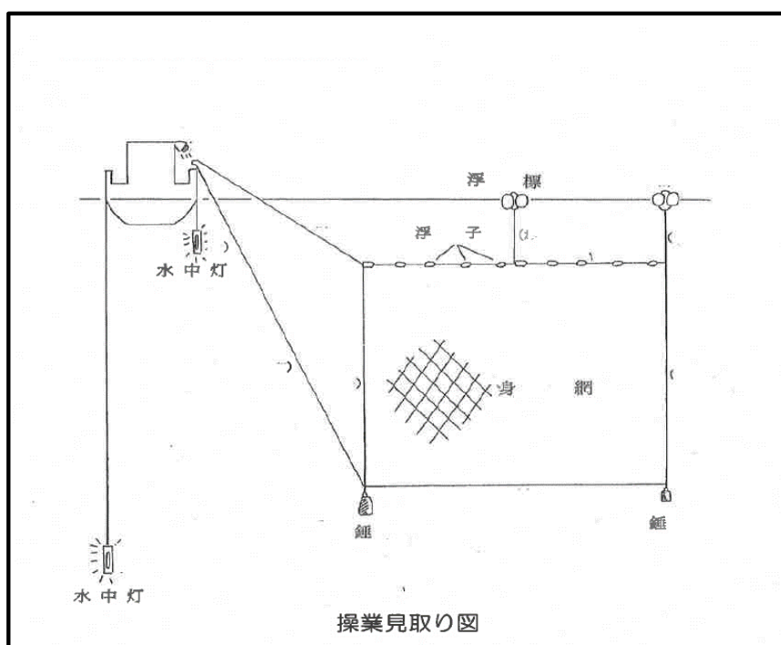
きびなさし網漁業漁法図
