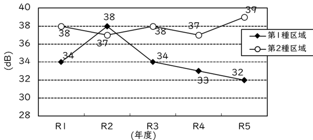
図 2-2 振動レベル ( L_{10} ) の経年変化（昼間）
