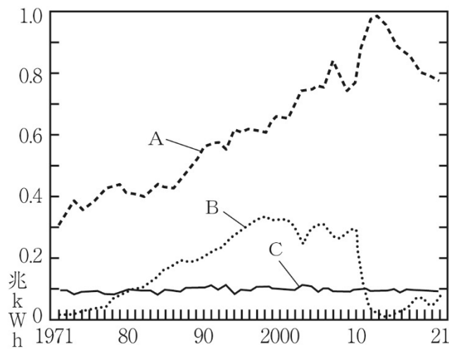
発電電力量の推移（会計年度）
