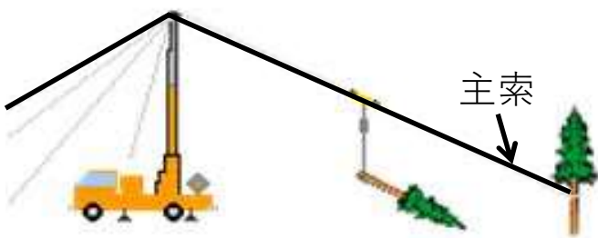
ｸﾞｰﾔｰﾀﾞ で主索を設置しての集材
