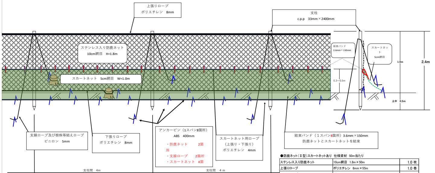
防鹿ネット（II型） 後付けネット型 標準図
