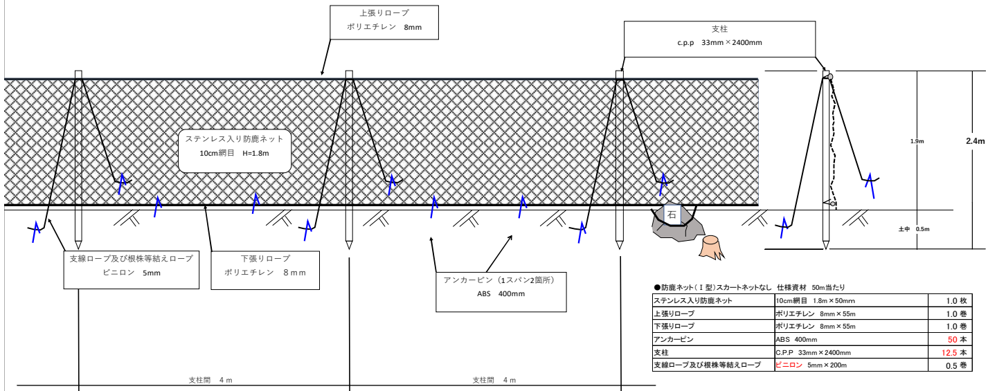
防鹿ネット（I型） 後付ネット無型 標準図
