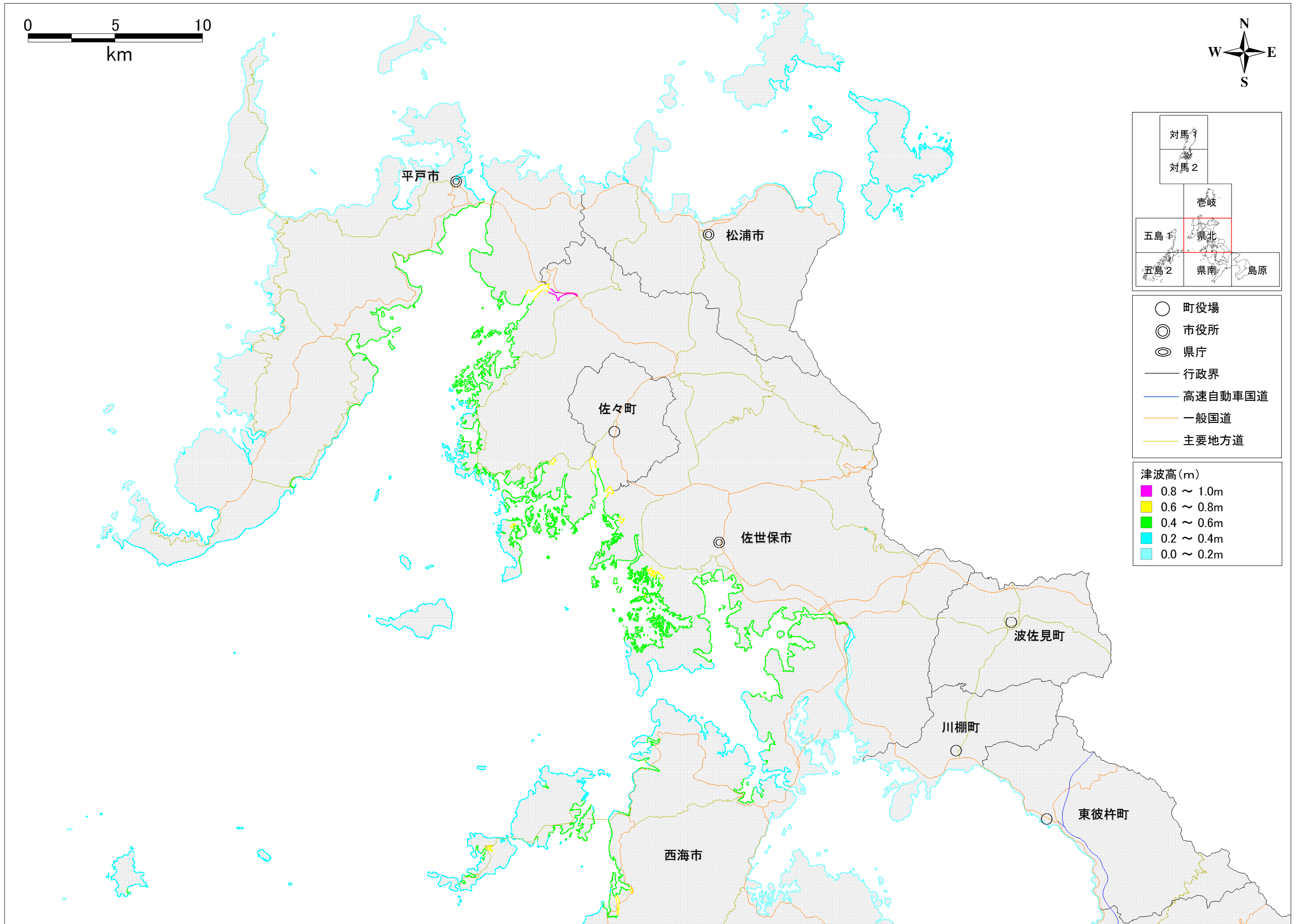
最大津波高分布図 県北（初期潮位=既往最大潮位 堤防等施設が機能する場合）
