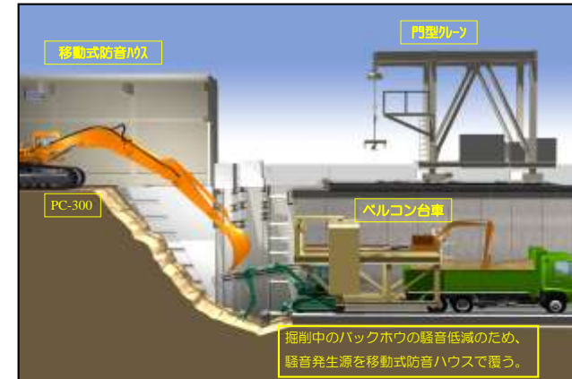
(施工設備配置状況CG)
