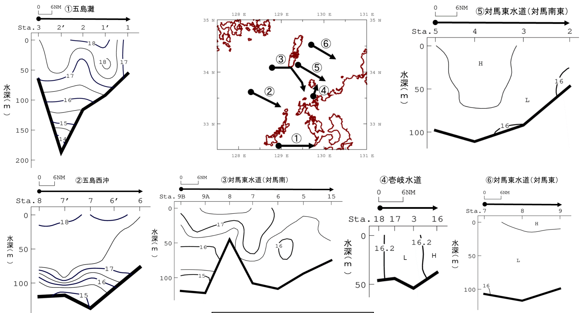
図1 水温鉛直断面図
