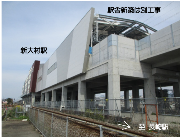
竣工した「新大村駅高架橋他」工区 (新大村駅部)
