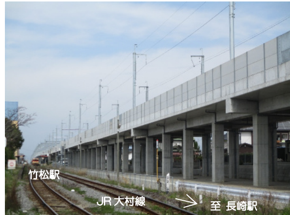
竣工した「新大村駅高架橋他」工区 (竹松駅付近)
