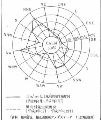
風向風速図
