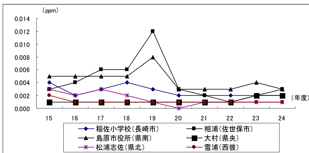
図2-2-1-7 二酸化硫黄の年平均値の経年変化
