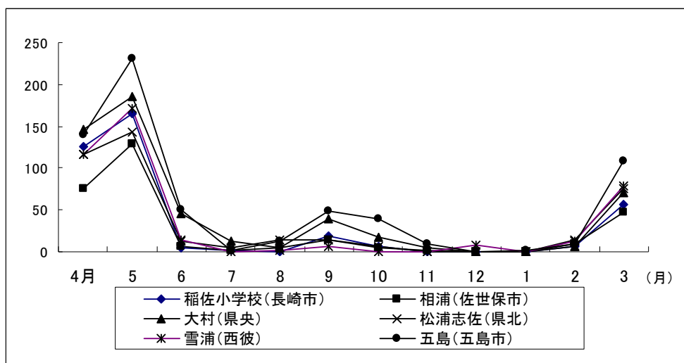
図2-2-1-18 光化学オキシダントの環境基準月別超過状況（平成24年度）
