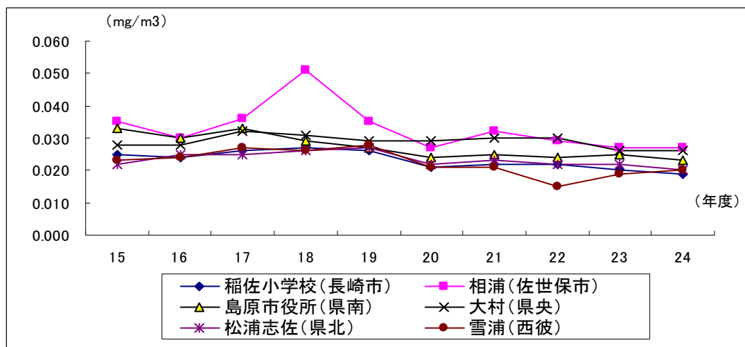
図2-2-1-11 浮遊粒子状物質の年平均値の経年変化
