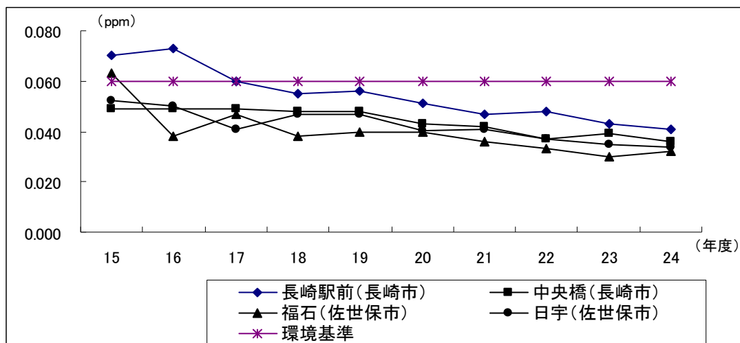
図2-2-2-1 二酸化窒素の98%値の経年変化
