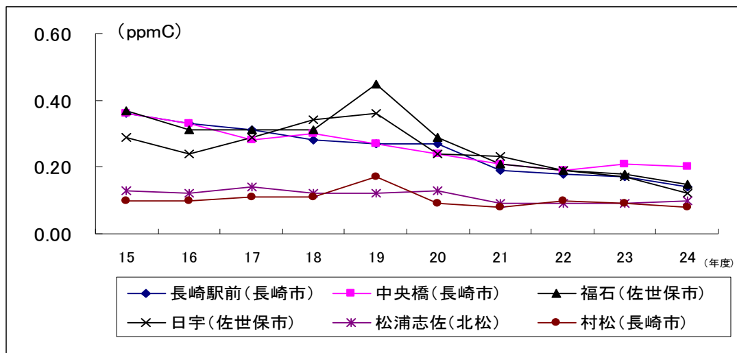
図2-2-1-22 非メタン炭化水素の年平均値の経年変化
