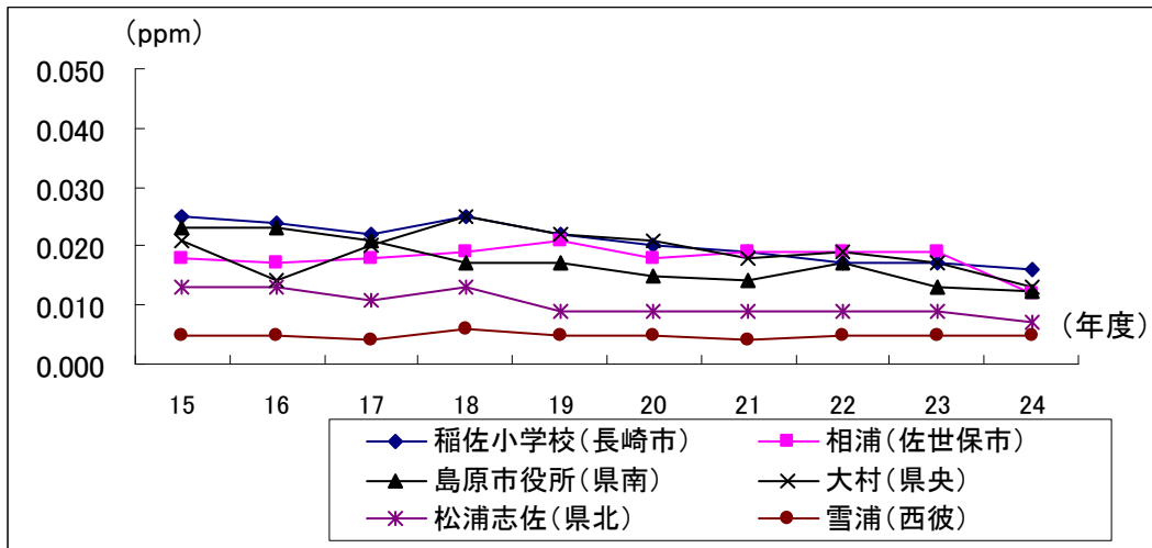
図2-2-1-14 二酸化窒素の98%値の経年変化
