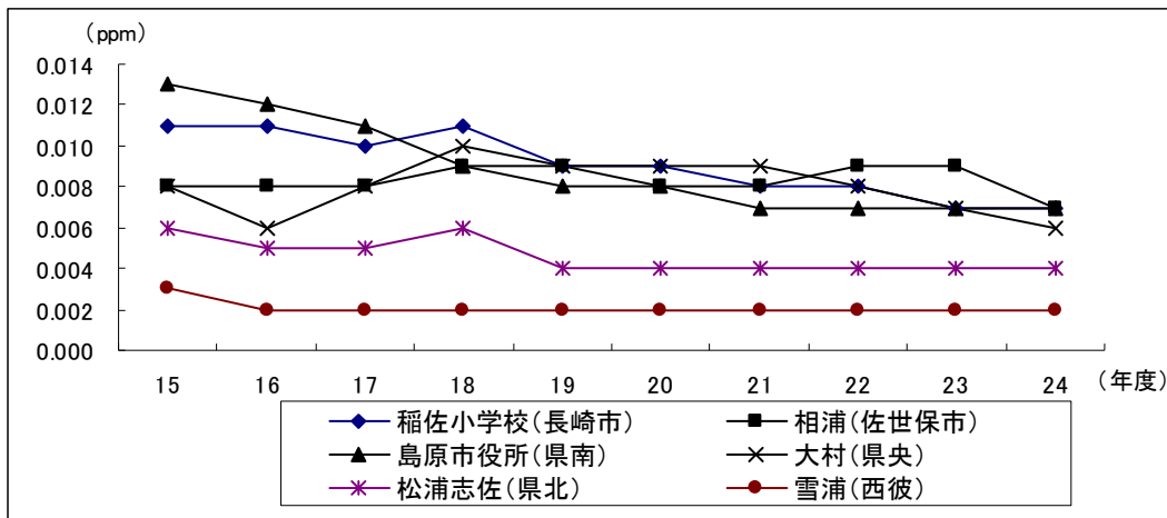
図2-2-1-15 二酸化窒素の年平均値の経年変化
