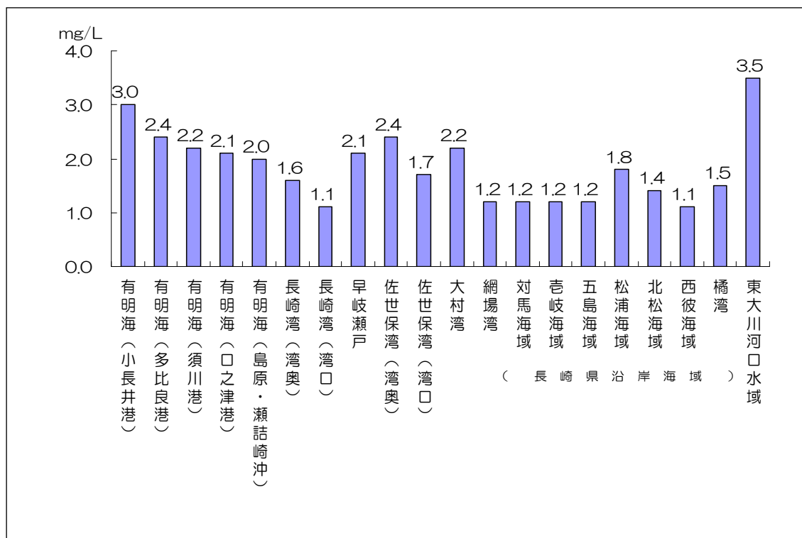
図2-3-1-4 平成24年度 海域のCOD75%値
