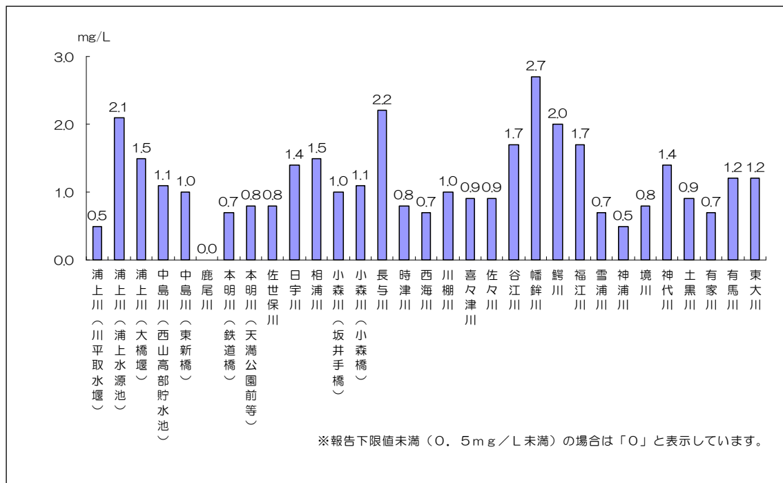
図2-3-1-2 平成24年度 主要河川のBOD75%値
