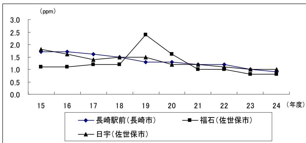
図2-2-2-2 一酸化炭素の2%除外値の経年変化
