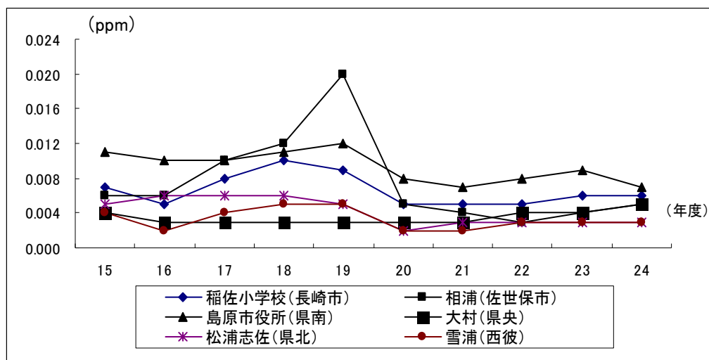
図2-2-1-6 二酸化硫黄の2%除外値の経年変化
