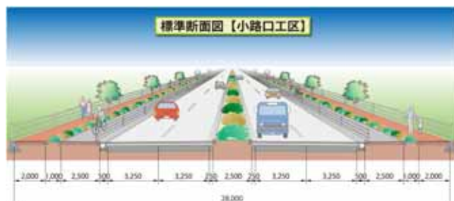
池田沖田線【小路口工区】 標準断面図
