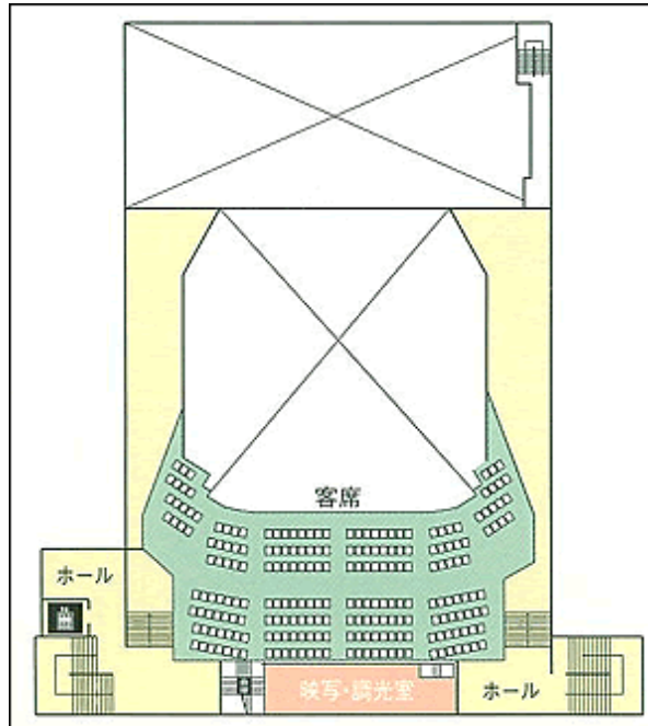
平面図(3F)
