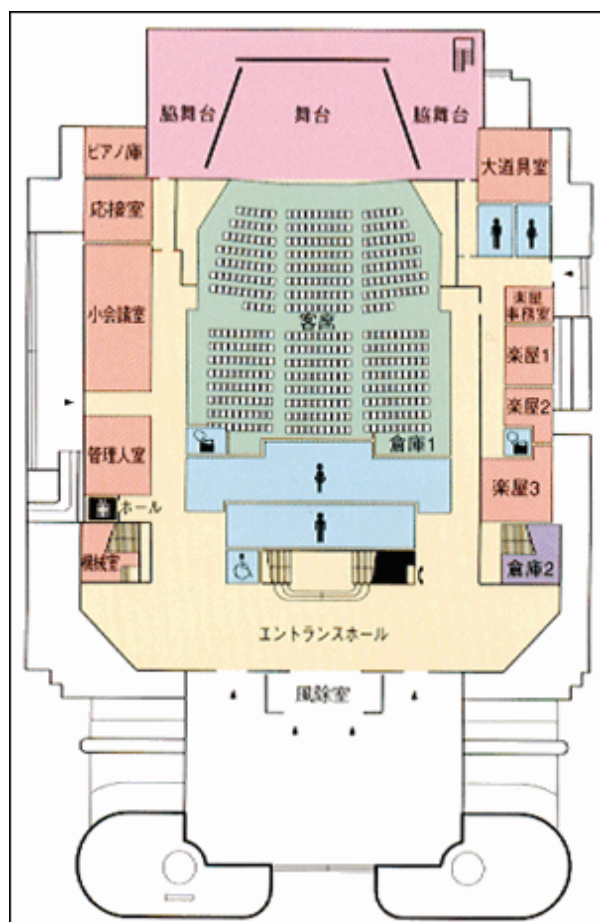
平面図(1F)
