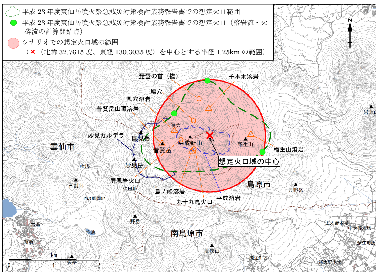
図12 想定火口域の範囲（国土地理院発行の『基盤地図情報』『基盤地図情報（数値標高モデル）』を使用した）
