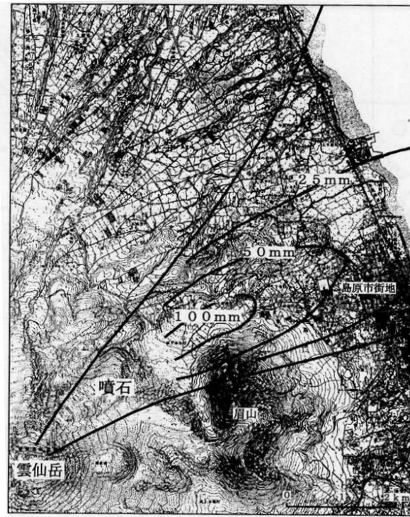
図 10 1991 年 6 月 11 日の爆発的噴火に伴う降灰分布図(気象庁, 2002) 国土地理院 1/25,000 地形図「雲仙」(昭和 60 年 1 月 30 日発行) による。
