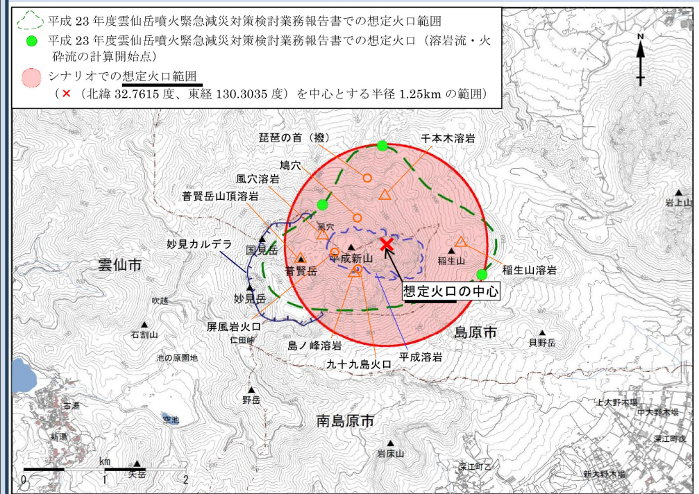
図12 想定火口範囲
