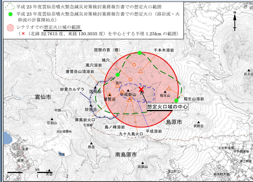
図12 想定火口域の範囲
