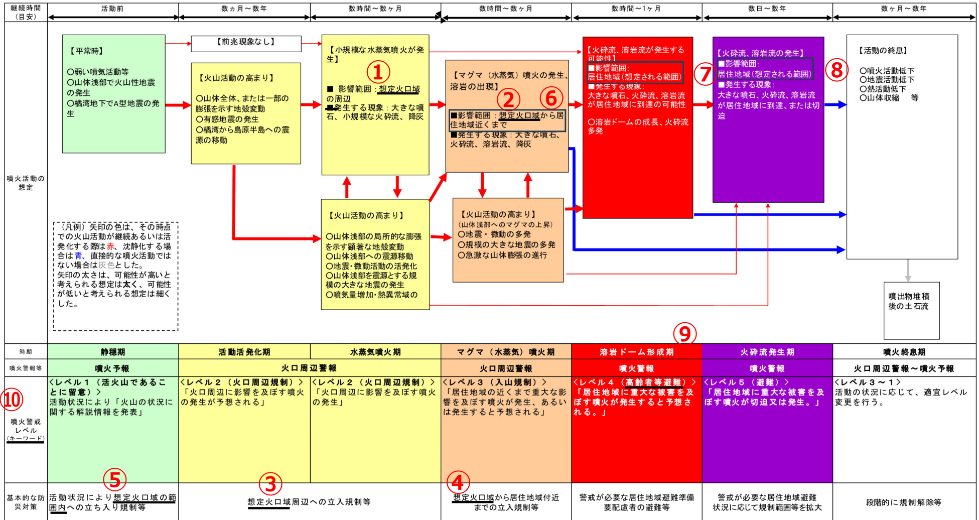
図 18 シナリオ 2 における火山活動の推移
