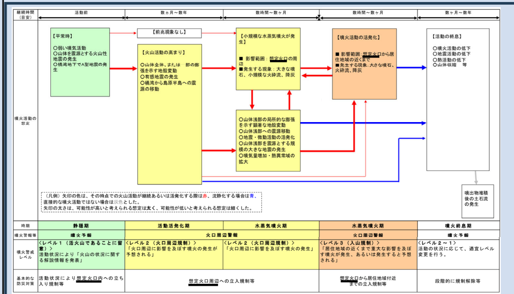
図17 シナリオ 1 における火山活動の推移
