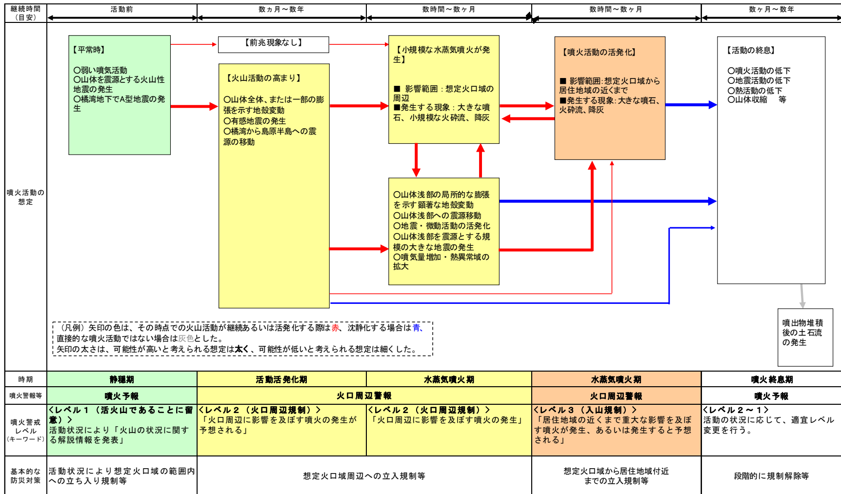
図 17 シナリオ 1 における火山活動の推移
