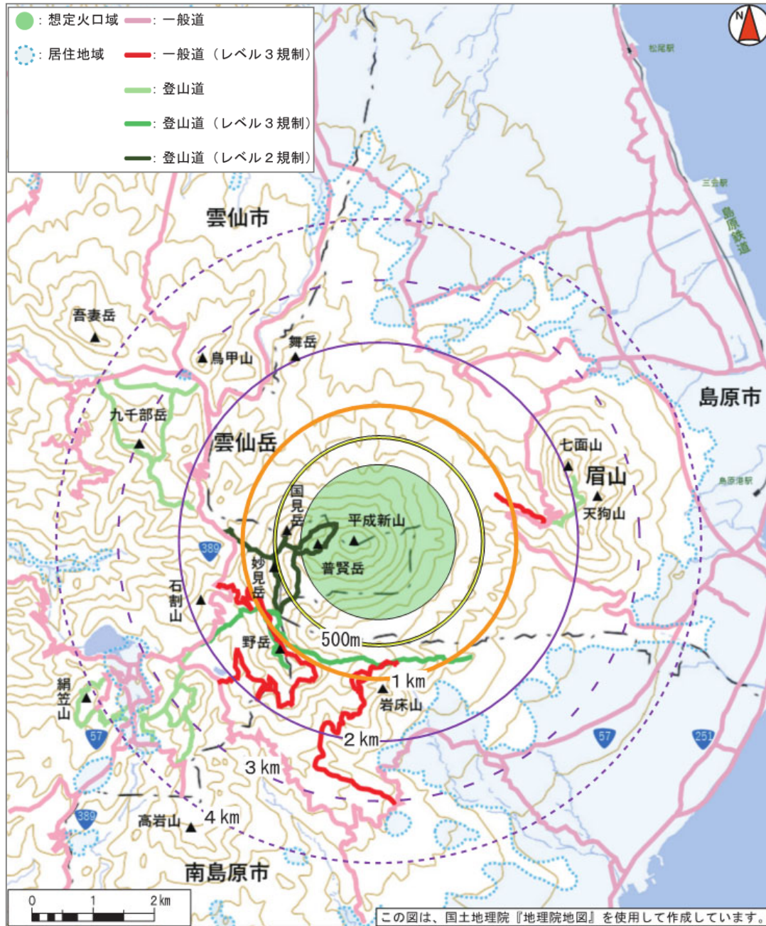
図13 想定火口域からの大きな噴石の影響範囲
