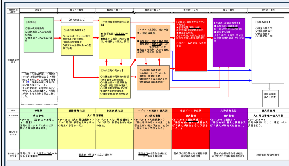
図18 シナリオ 2 における火山活動の推移
