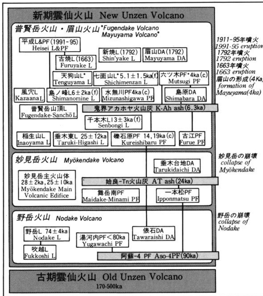
図3 雲仙岳の層序関係図 (渡辺・星住, 1995)
