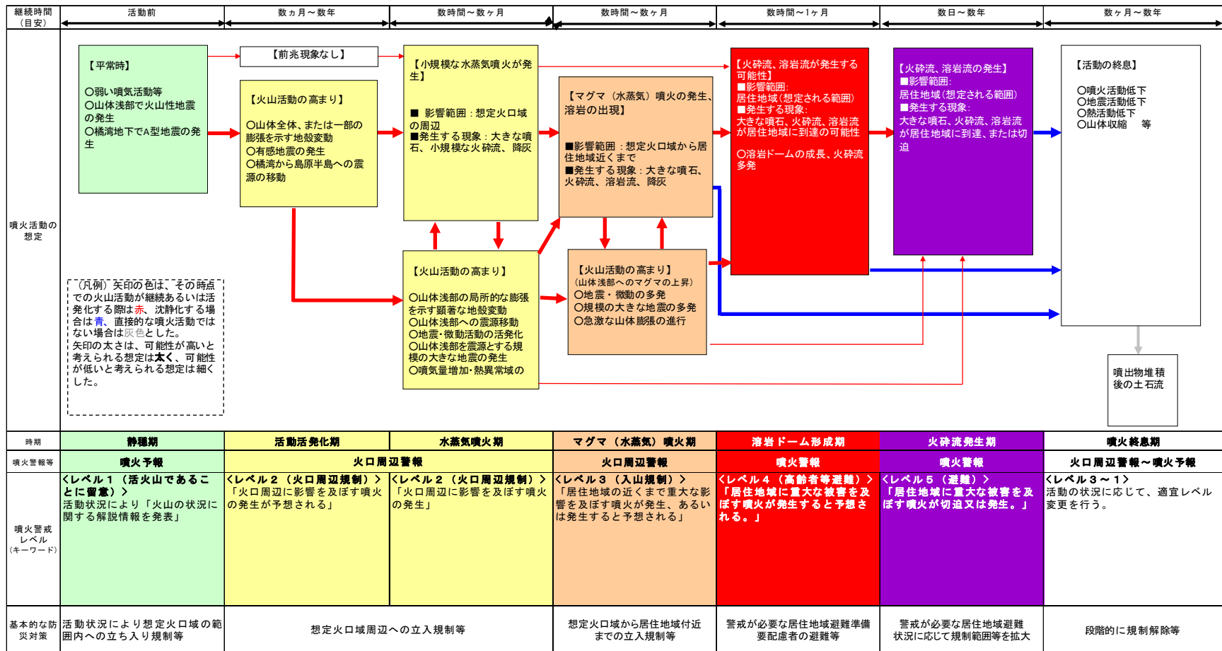
図 18 シナリオ 2 における火山活動の推移
