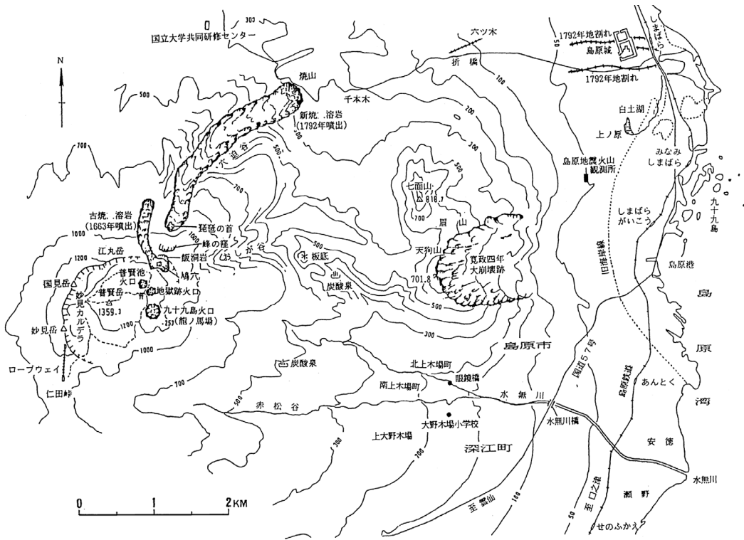
図4 1663年古焼溶岩、1792年新焼溶岩(太田, 1985)
