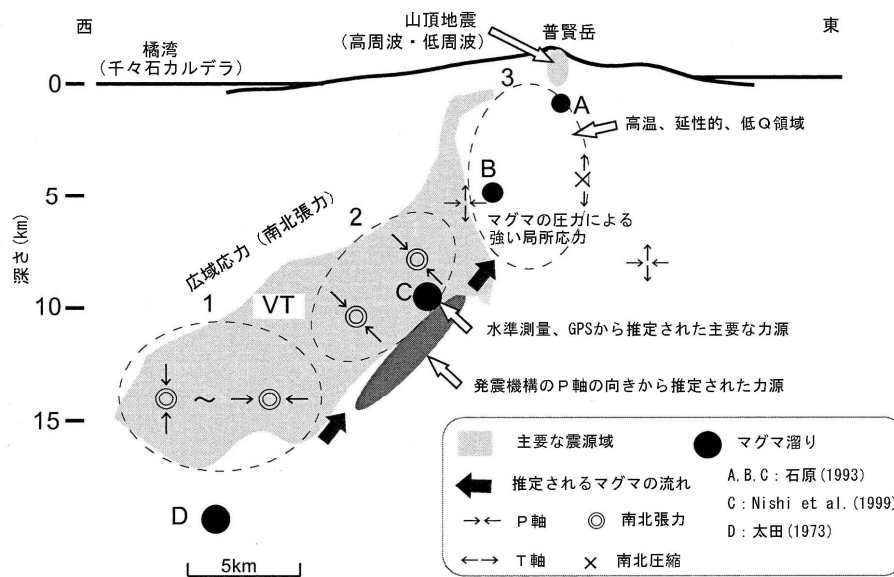
図8 1990～1996年雲仙岳噴火活動のマグマ上昇経路 (Umakoshi et al., 2001 を翻訳)
