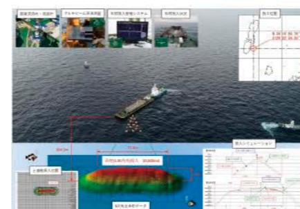
工事名 対馬東方地区マウンド礁整備工事 施工業者 大石・小宮特定建設工事共同企業体 技術者 原 拓也
