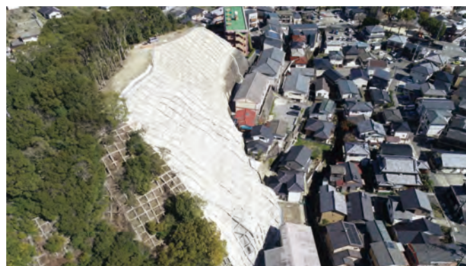
令和7年度概成 金堀(1)地区急傾斜地崩壊対策事業（長崎市）
