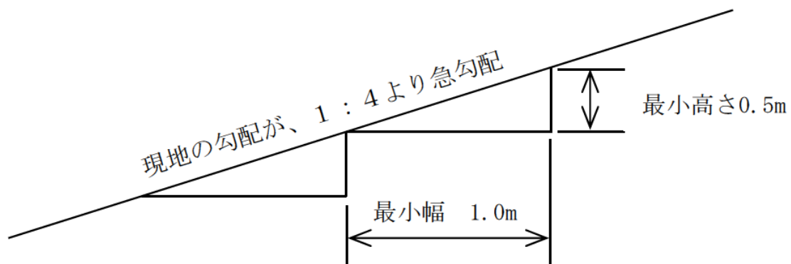
図4-1 盛土基礎地盤の段切
