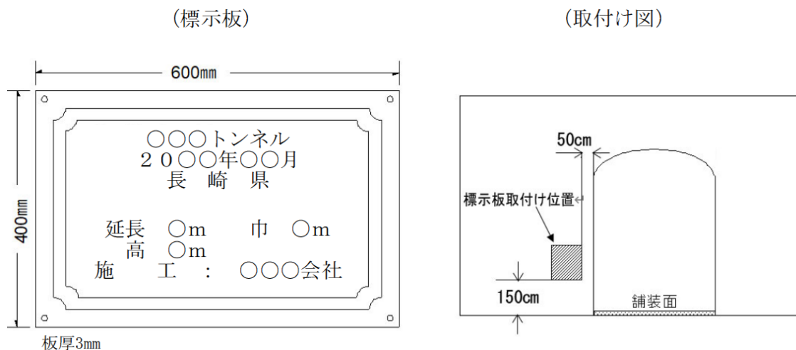
図 6-2 表示板の設置イメージ図
