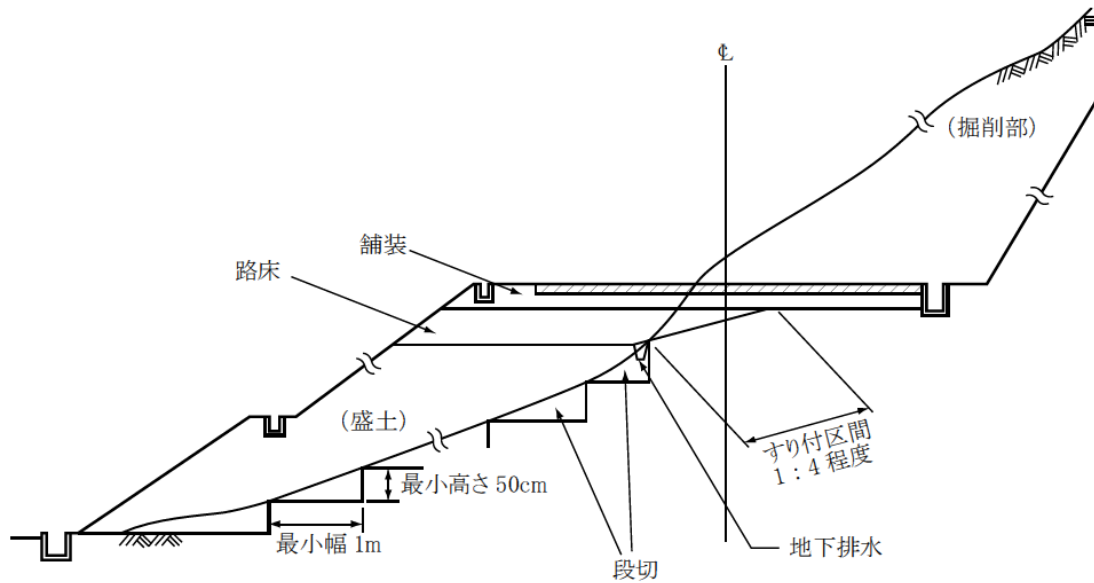
図 4 - 2 盛土基礎地盤の段切
