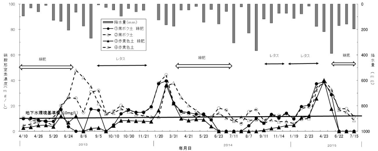
図1 試験期間中の降水量(mm)と浸透水中の硝酸態窒素濃度(mg/L)の推移
