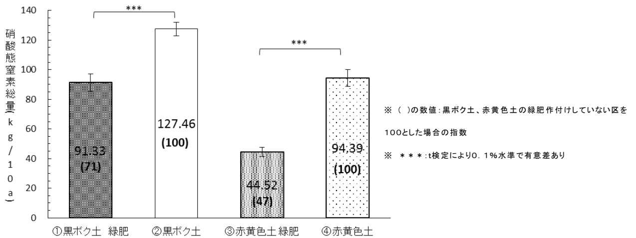
図2 試験期間中の浸透水中の硝酸態窒素総量(kg/10a)
