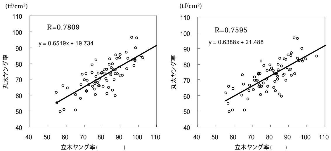
図2 丸太と立木のヤング率
