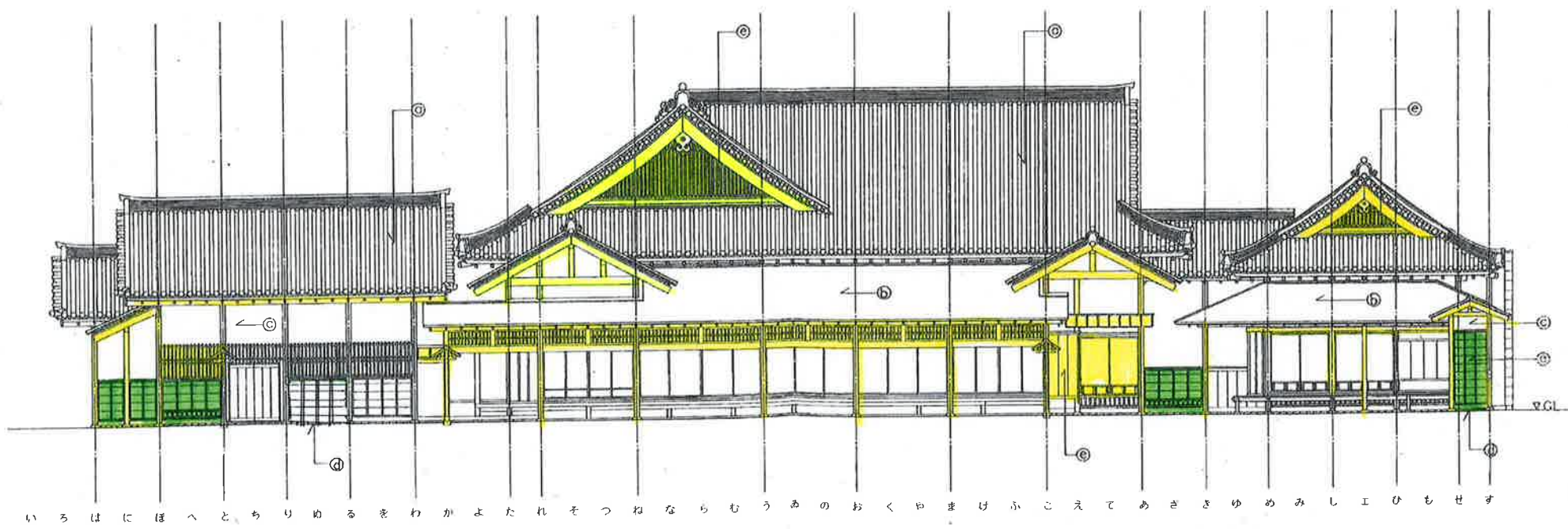
東側立面図
