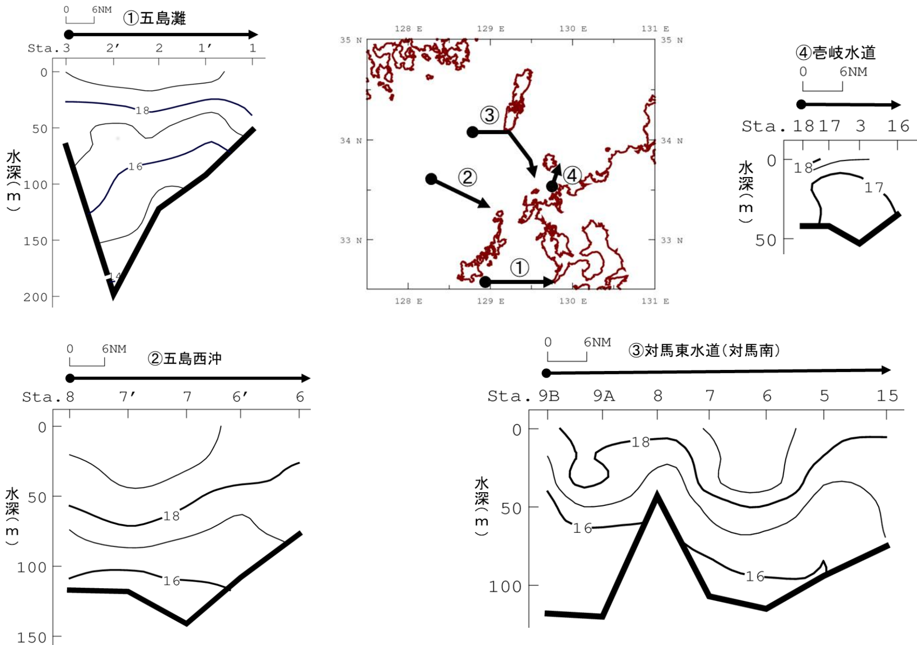
図1 水温鉛直断面図
