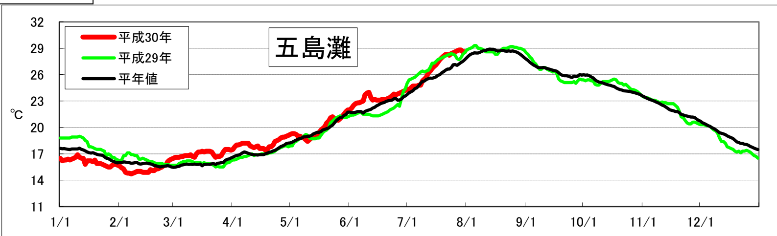
図2 長崎県周辺海域の海面水温の推移
