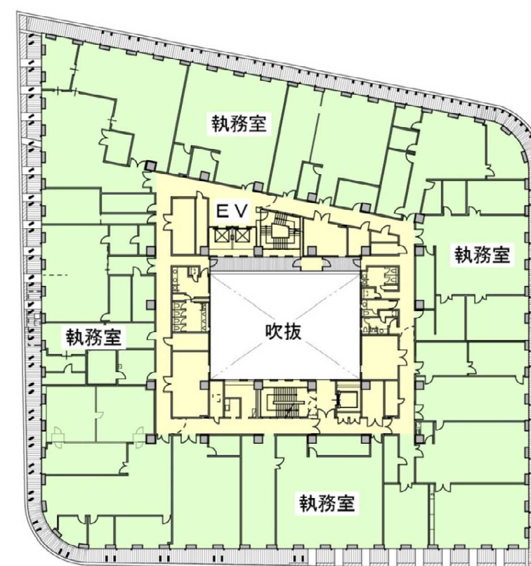
5階 平面図
