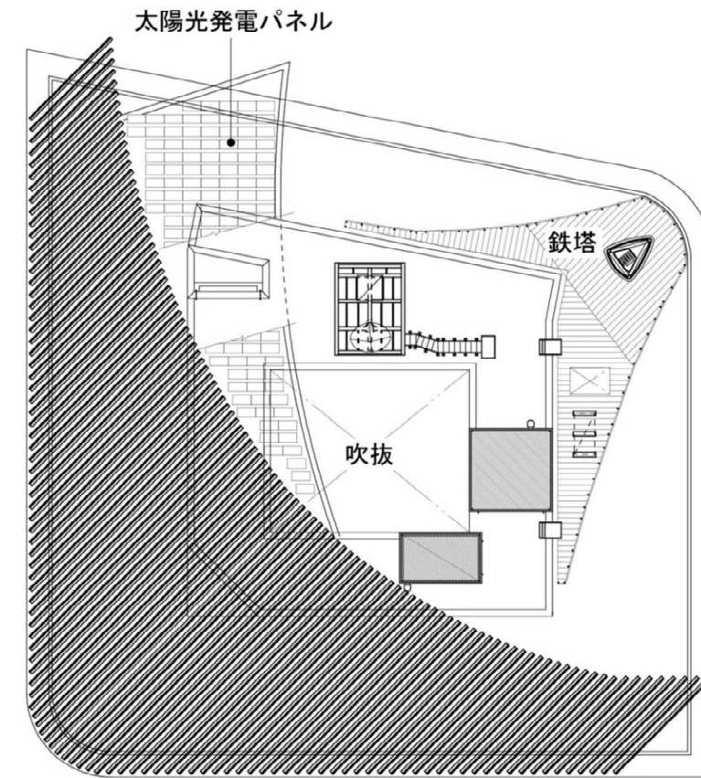
R階 平面図
