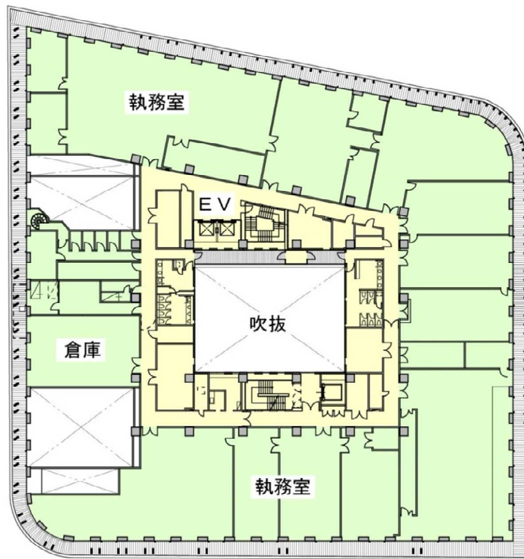
7階 平面図
