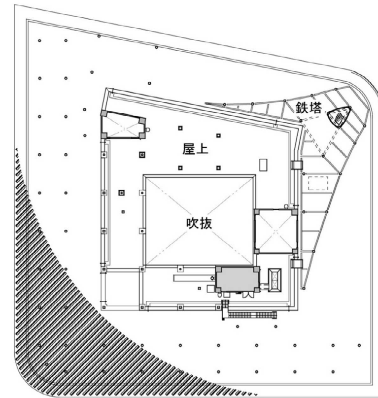
PH階 平面図
