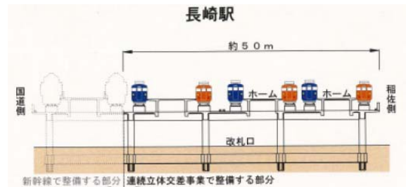
図-12 長崎駅の構造
