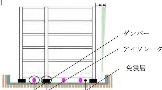
<免震構造のイメージ図>
